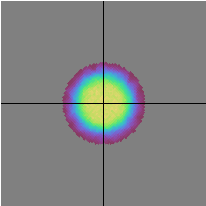
baseline_v2.1_10yrs y band: DD:ECDFS NVisits
