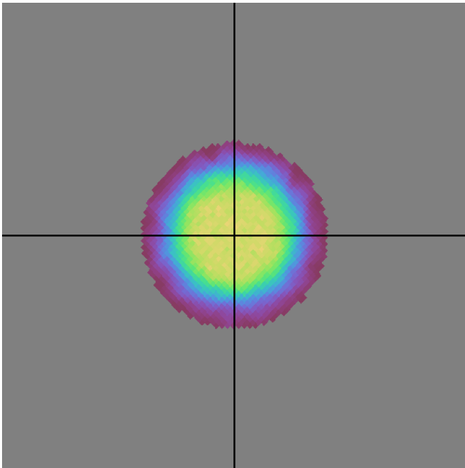
baseline_v2.1_10yrs i band: DD:ECDFS NVisits
