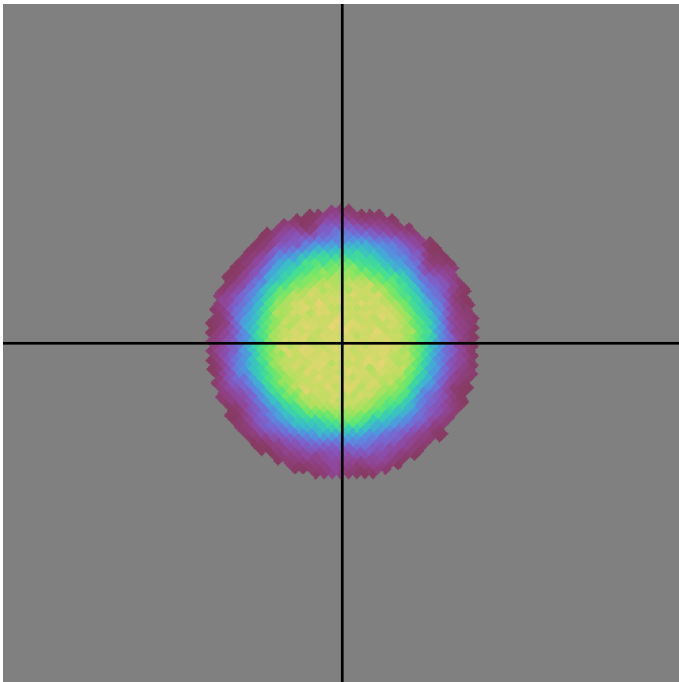
baseline_v2.1_10yrs g band: DD:ECDFS NVisits
