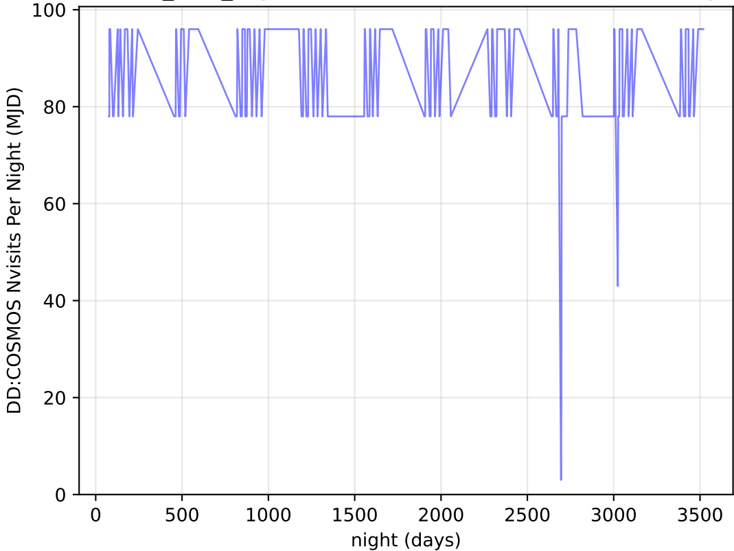
baseline_v2.1_10yrs all bands: DD: COSMOS Nvisits Per Night
