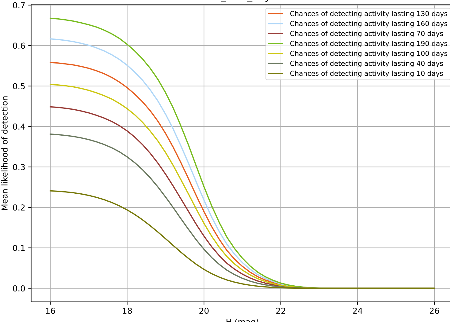
baseline v2.0 10yrs MBA
