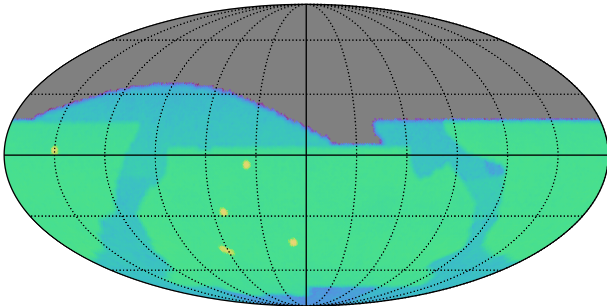
baseline_v2.0_10yrs i: SurfaceBrightLimit
