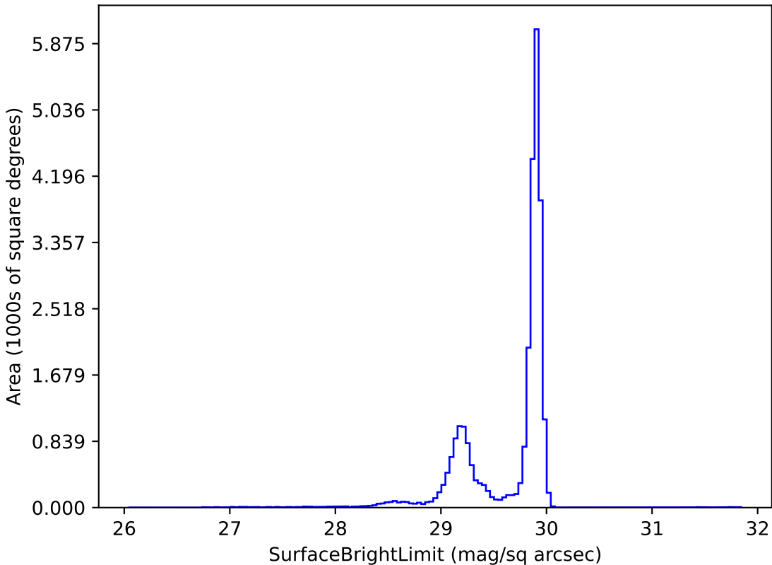
baseline_v2.0_10yrs i: SurfaceBrightLimit
