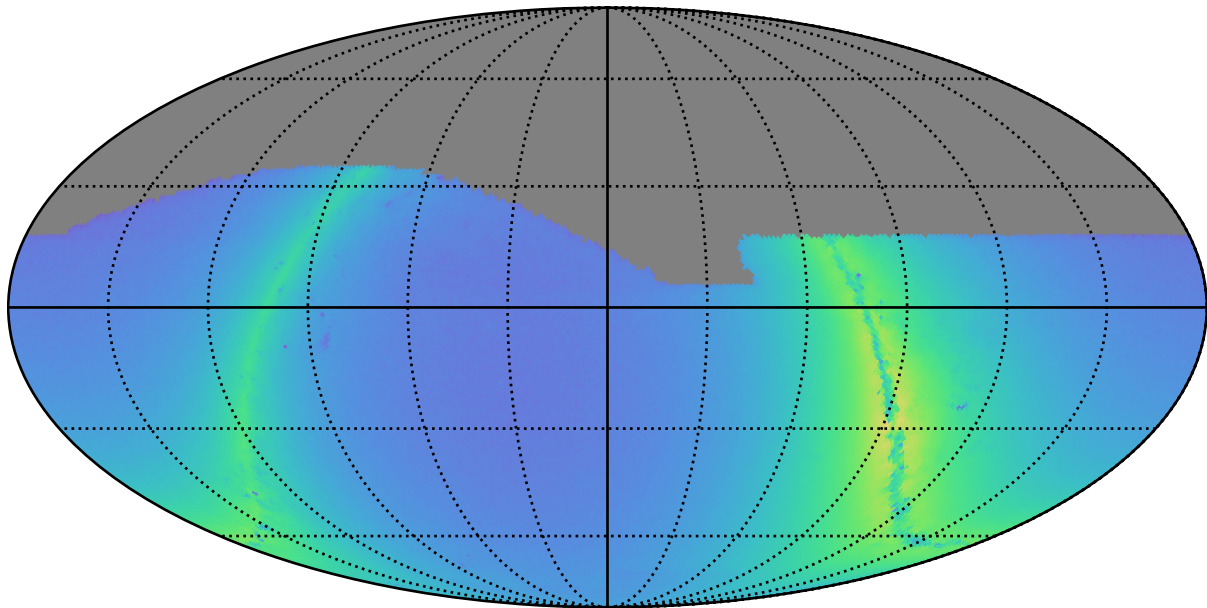
baseline_v2.0_10yrs i: Nstars_no_crowding
