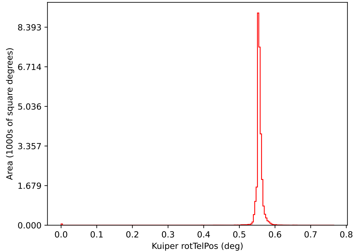
baseline_v2.0_10yrs i: Kuiper rotTelPos
