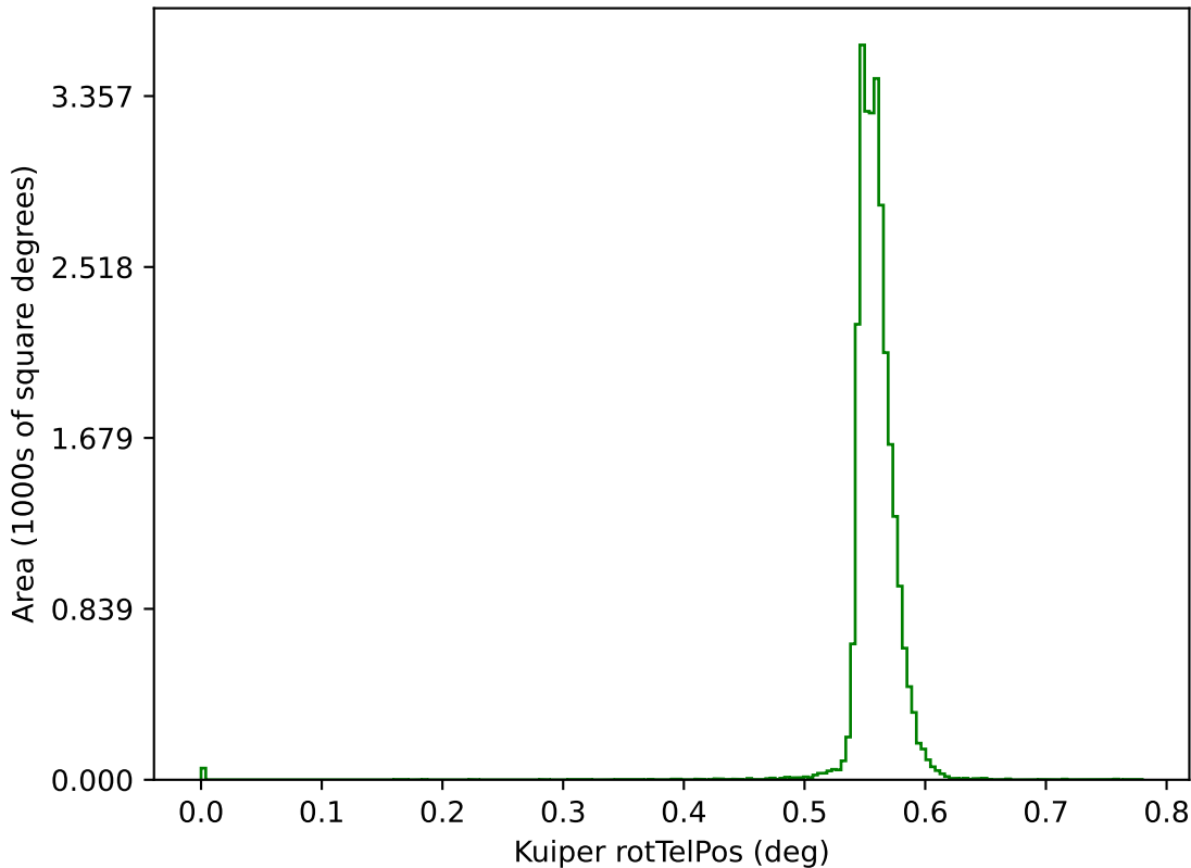
baseline_v2.0_10yrs g: Kuiper rotTelPos
