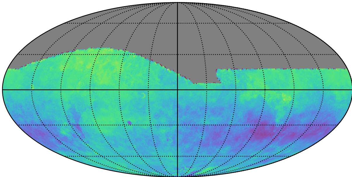
baseline_v2.0_10yrs z: Kuiper rotSkyPos
