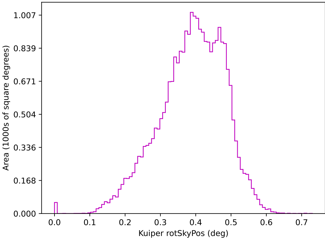
baseline_v2.0_10yrs z: Kuiper rotSkyPos
