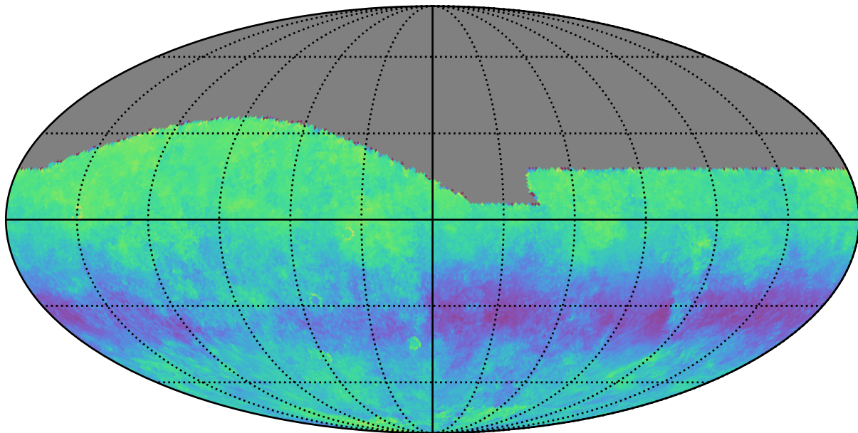
baseline_v2.0_10yrs g: Kuiper rotSkyPos
