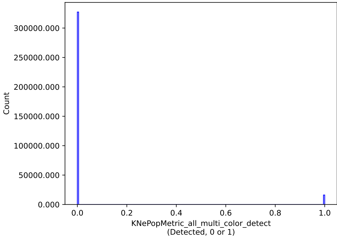
baseline_v2.0_10yrs all models: KNePopMetric_all_multi_color_detect
