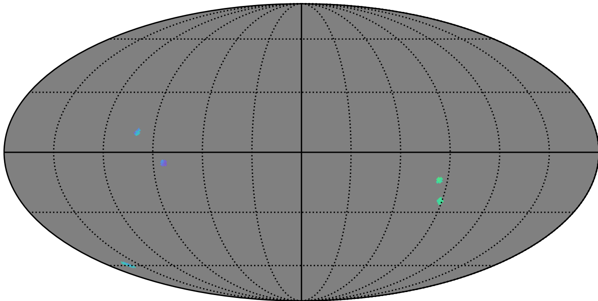
baseline_v2.0_10yrs : GalplaneTimePerFilter_bonito_sfr_map_g
