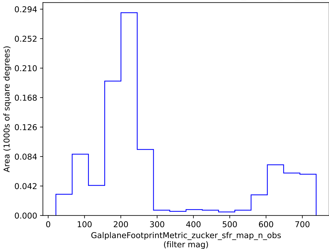
baseline_v2.0_10yrs : GalplaneFootprintMetric_zucker_sfr_map_n_obs
