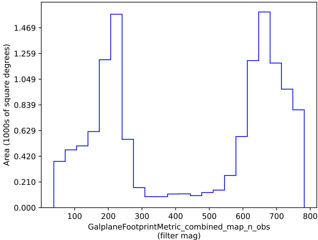
baseline_v2.0_10yrs : GalplaneFootprintMetric_combined_map_n_obs
