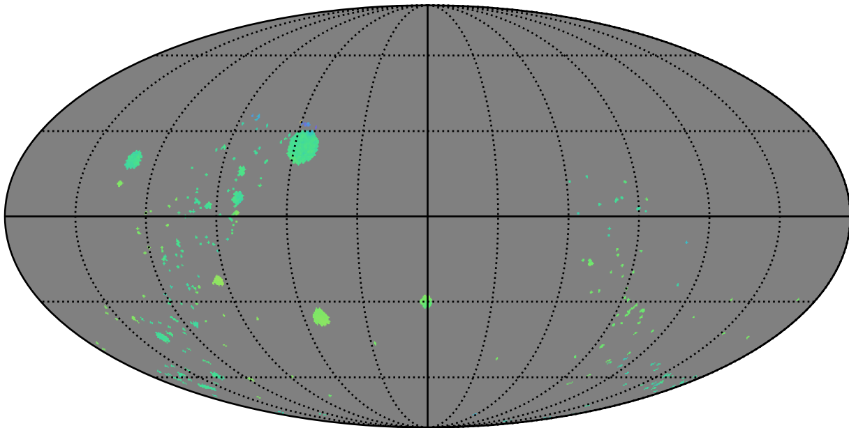
baseline_v2.0_10yrs : GalPlaneVisitIntervalsTimescales_open_clusters_map_Tau_2_0
