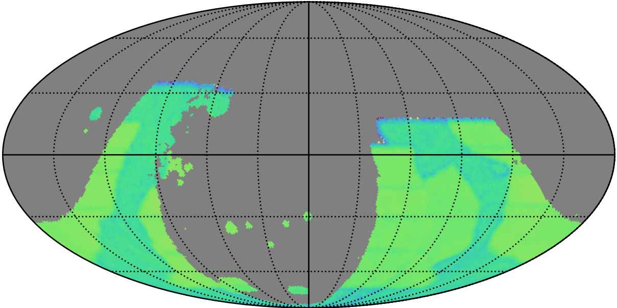
baseline_v2.0_10yrs : GalPlaneVisitIntervalsTimescales_combined_map_Tau_2_0
