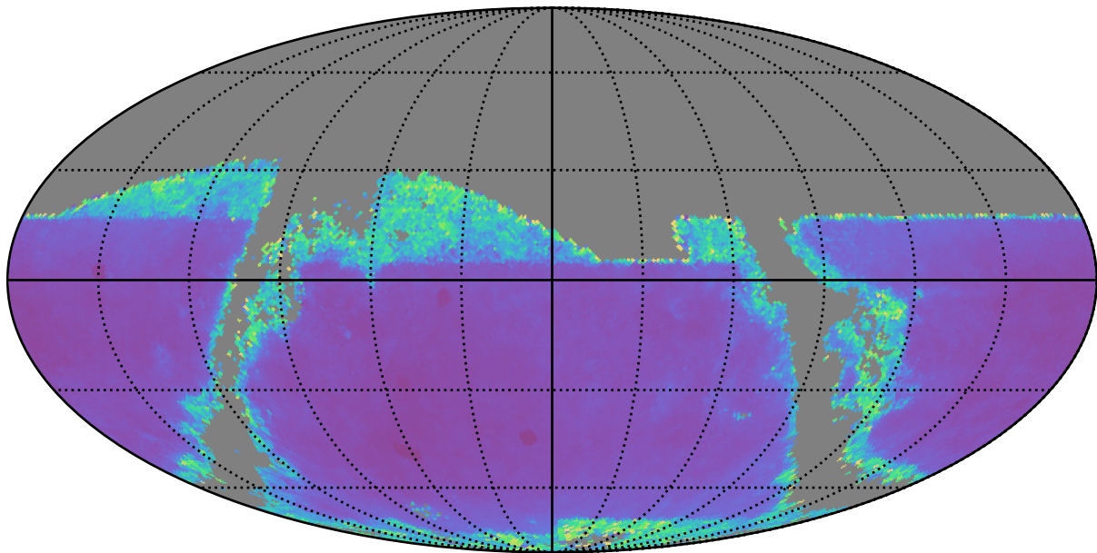
baseline_v2.0_10yrs z band: AGN SF_uncert
