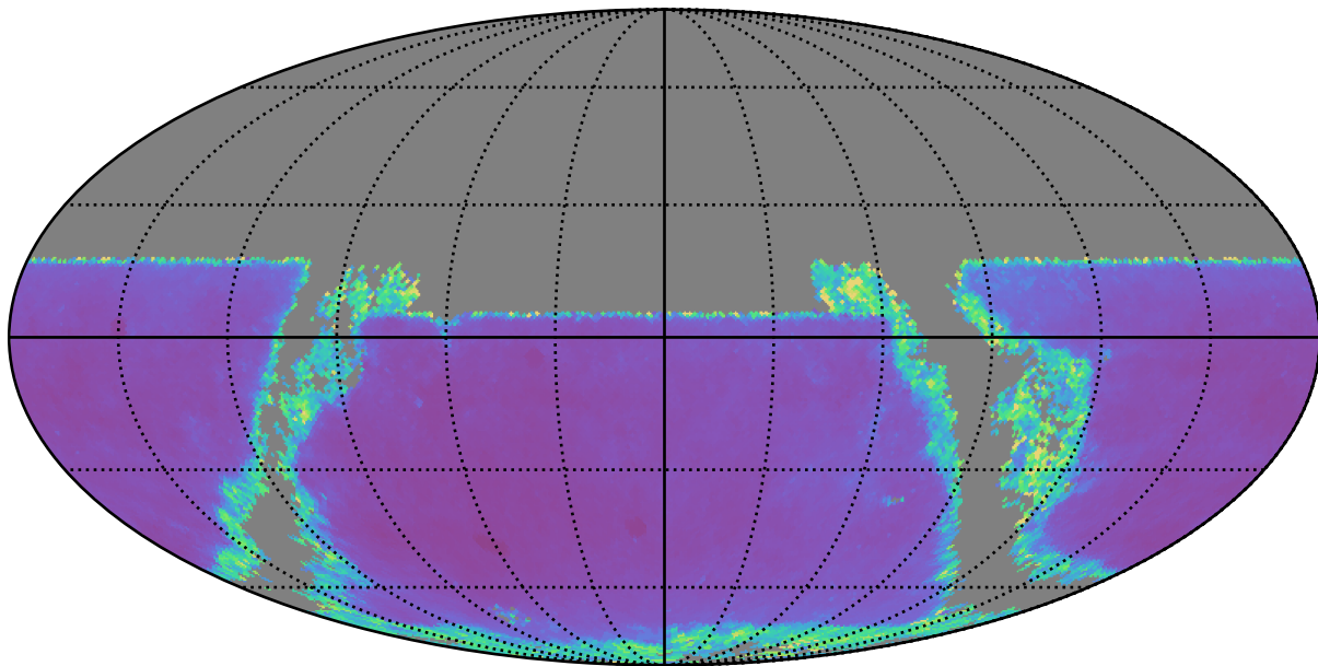
baseline_v2.0_10yrs y band: AGN SF_uncert
