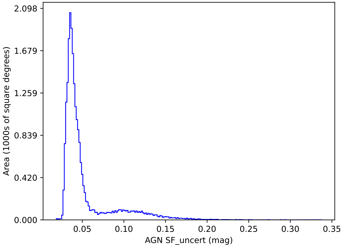
baseline_v2.0_10yrs y band: AGN SF_uncert
