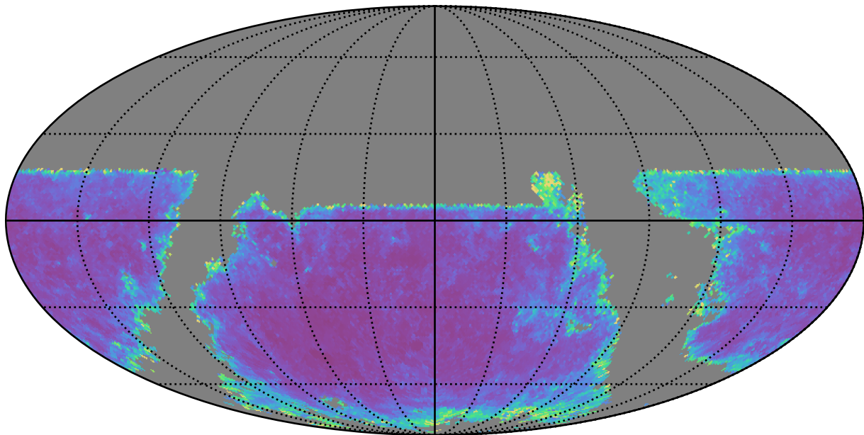
baseline_v2.0_10yrs u band: AGN SF_uncert
