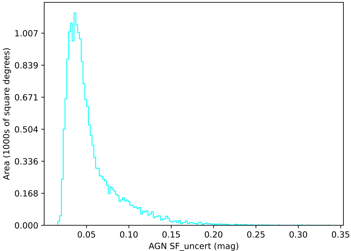
baseline_v2.0_10yrs u band: AGN SF_uncert
