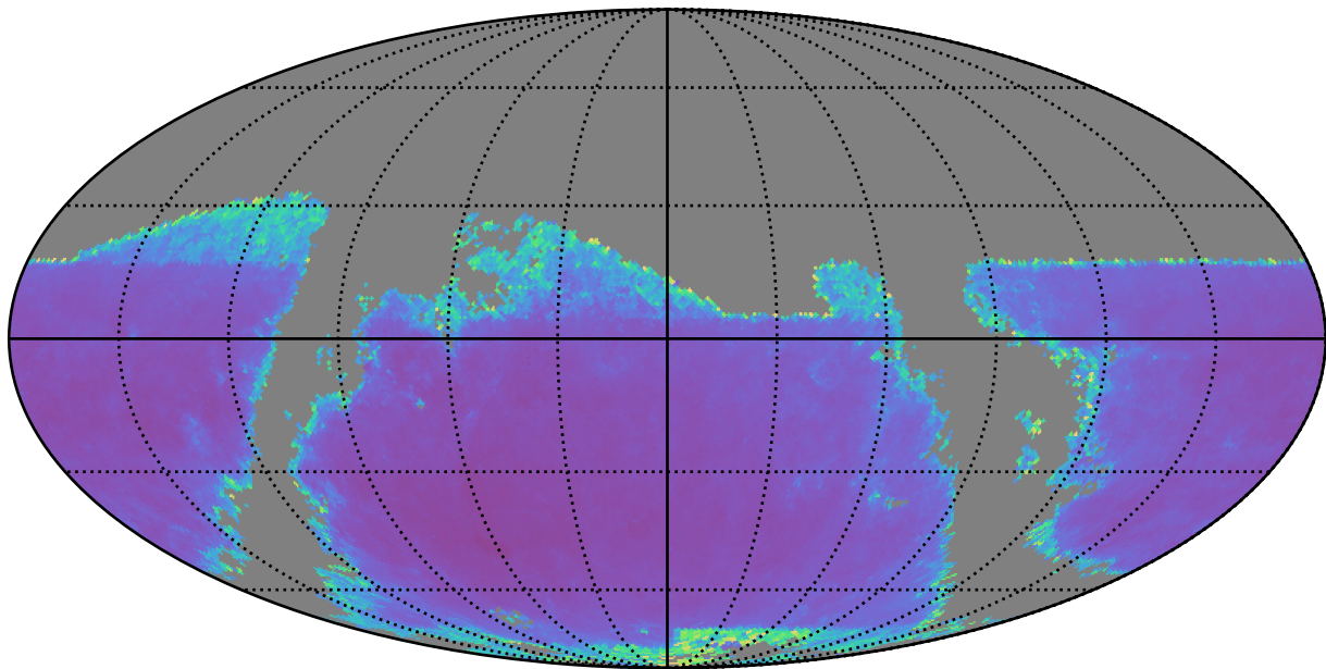
baseline_v2.0_10yrs r band: AGN SF_uncert
