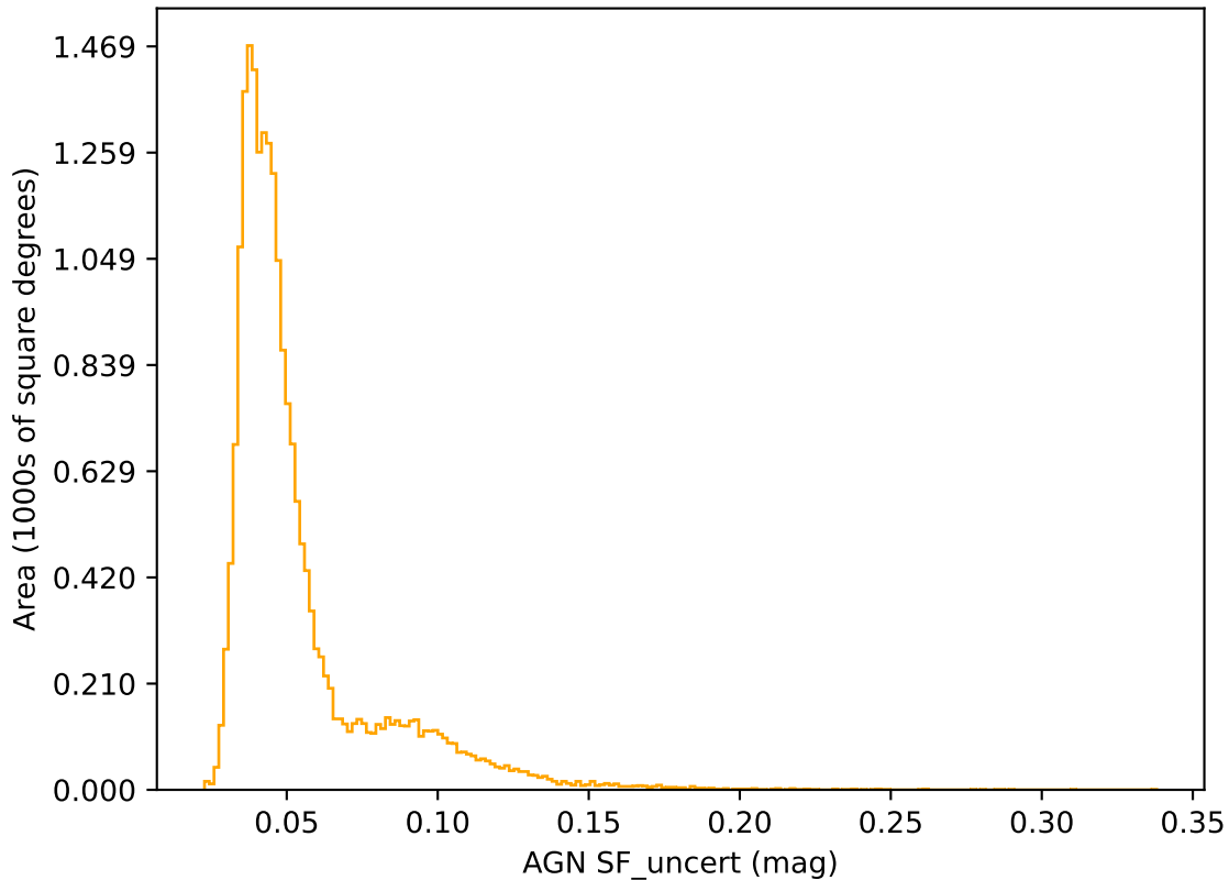
baseline_v2.0_10yrs r band: AGN SF_uncert
