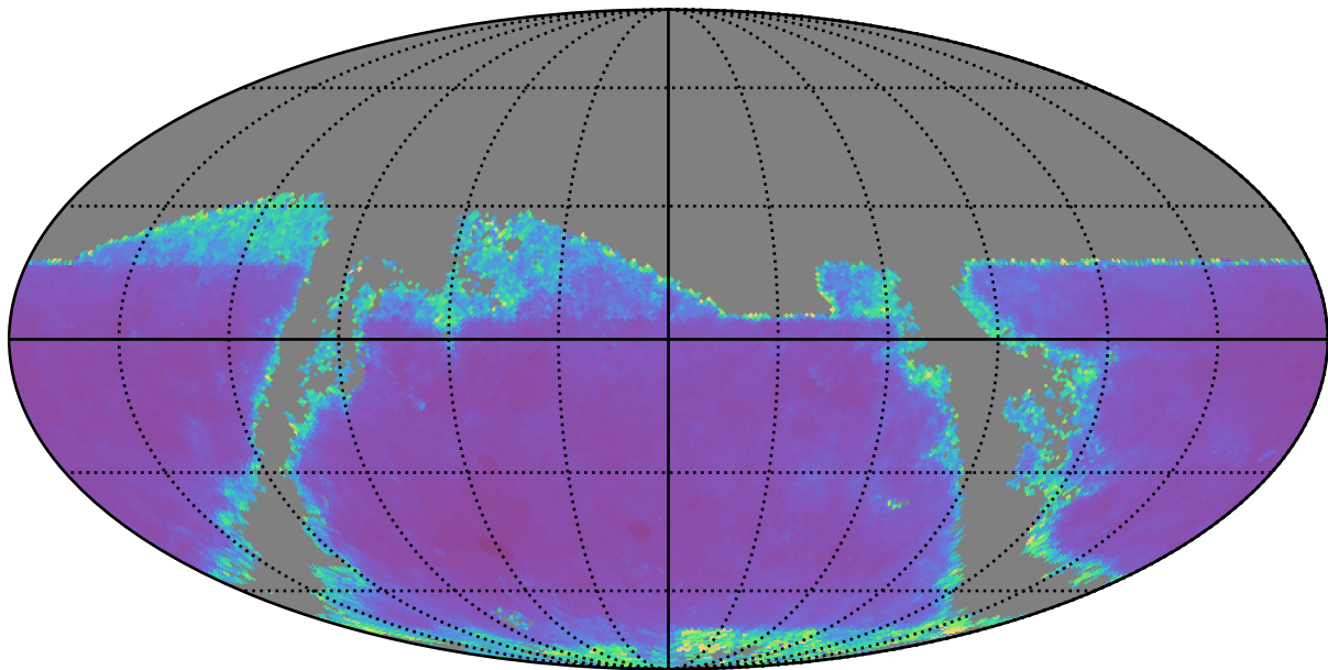
baseline_v2.0_10yrs i band: AGN SF_uncert
