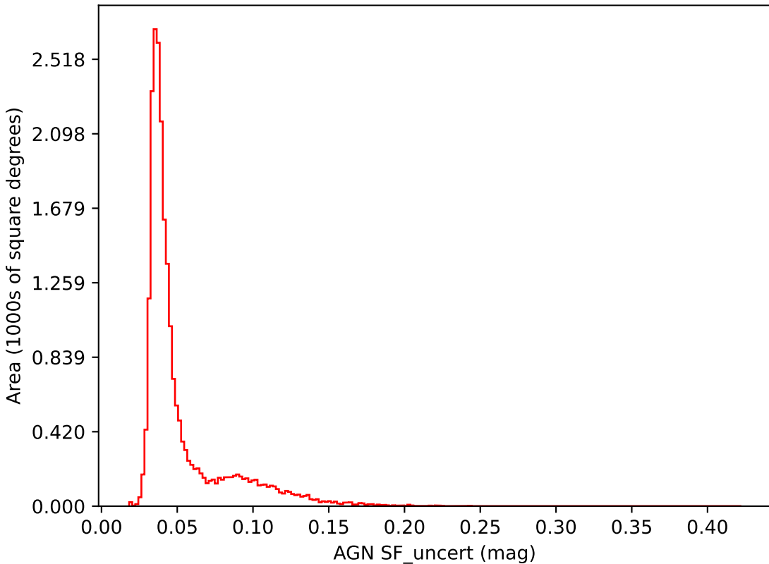
baseline_v2.0_10yrs i band: AGN SF_uncert
