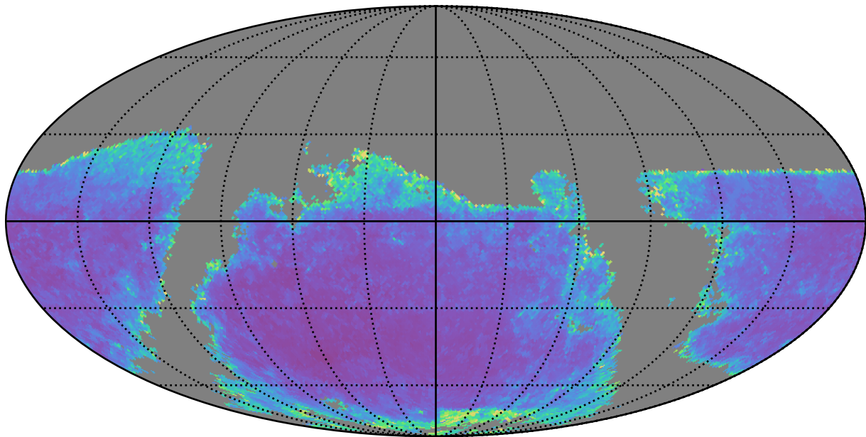
baseline_v2.0_10yrs g band: AGN SF_uncert
