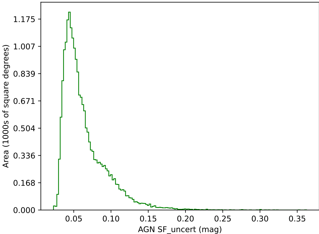
baseline_v2.0_10yrs g band: AGN SF_uncert
