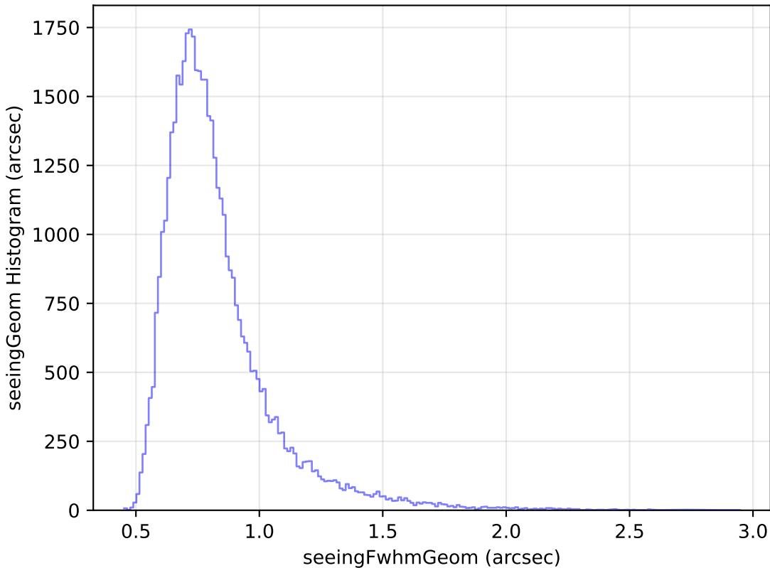
baseline_v2.0_10yrs Yr 1 y band: seeingGeom Histogram
