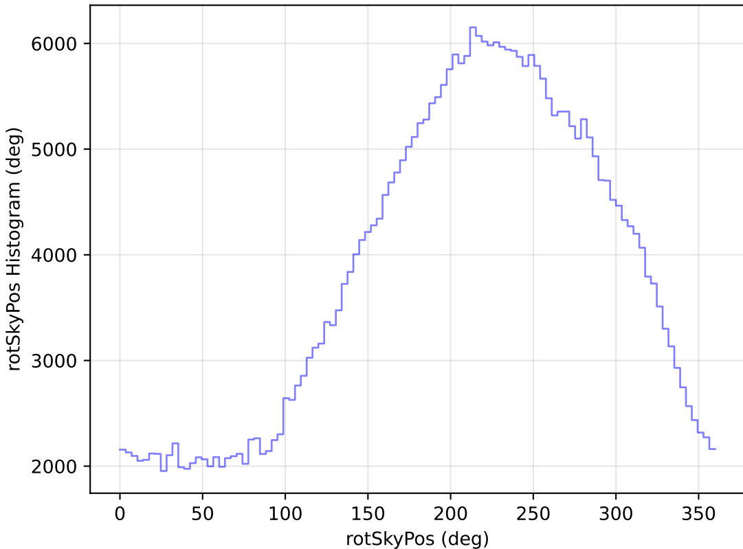
baseline_v2.0_10yrs WFD y band: rotSkyPos Histogram
