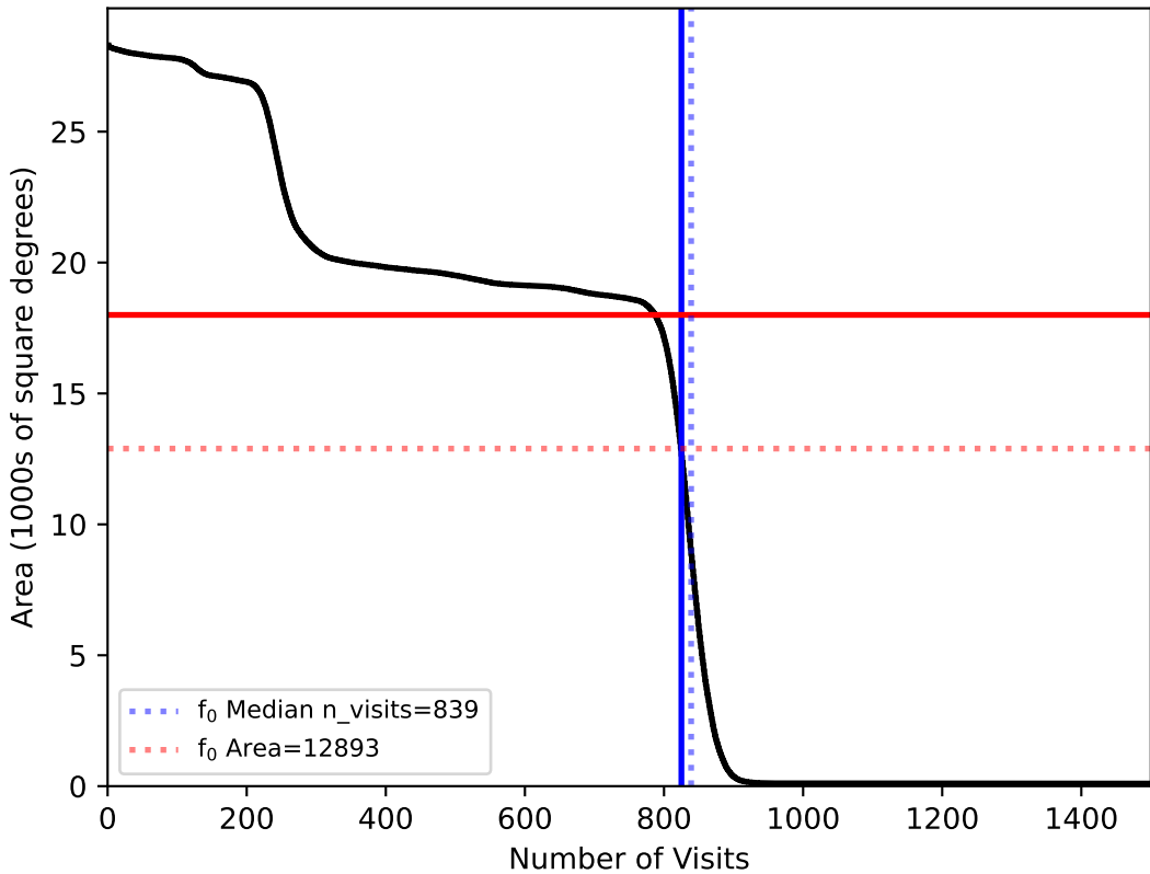
baseline_v2.0_10yrs All sky: f0
