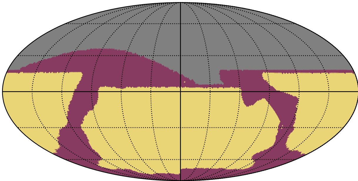
baseline_v2.0_10yrs All sky: RapidRevisits
