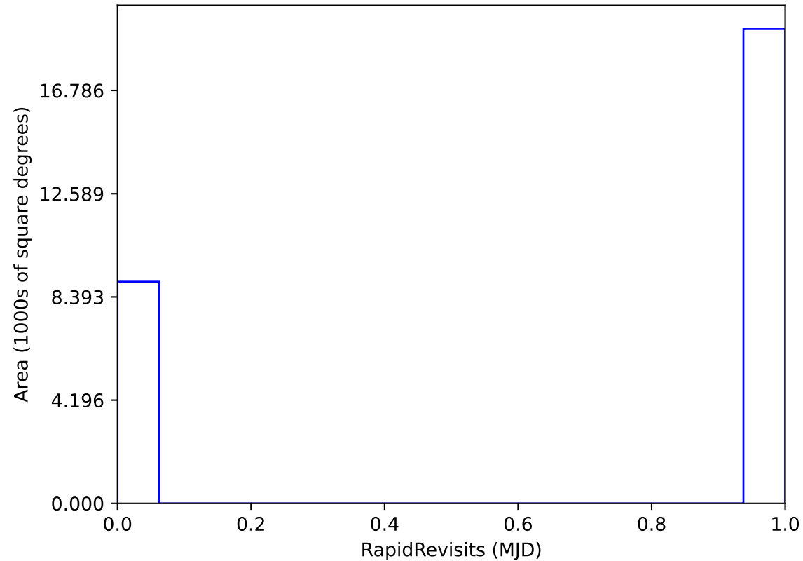
baseline_v2.0_10yrs All sky: RapidRevisits
