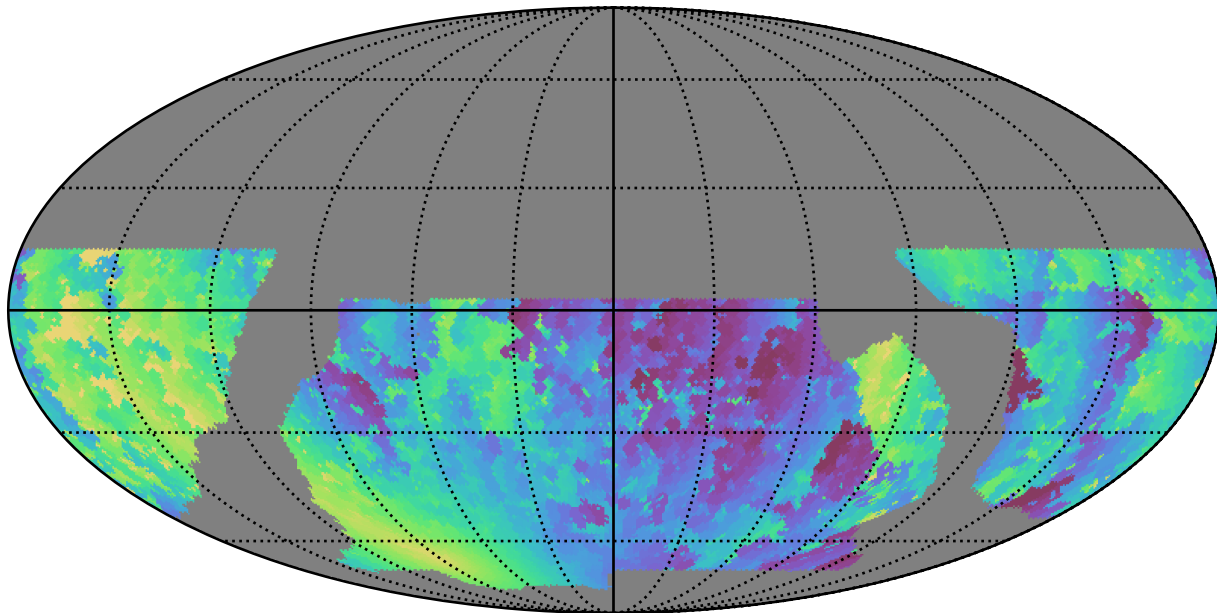
baseline_v2.0_10yrs WFD y band: Min solarElong
