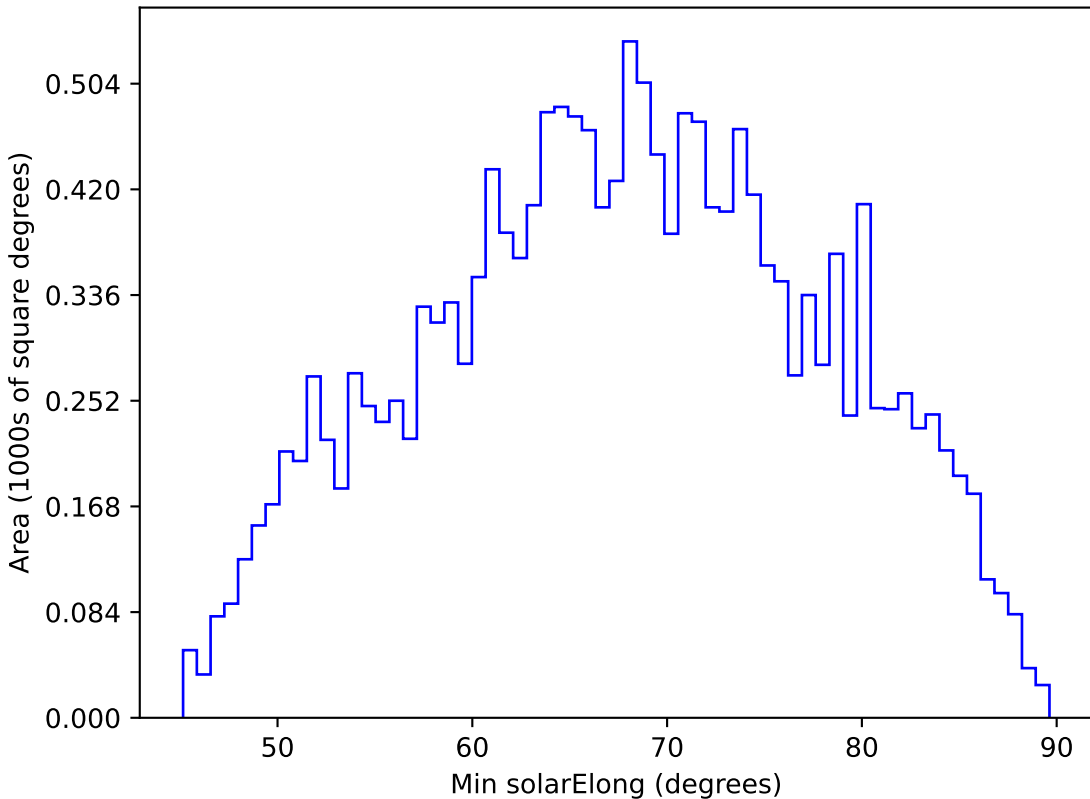
baseline_v2.0_10yrs WFD y band: Min solarElong
