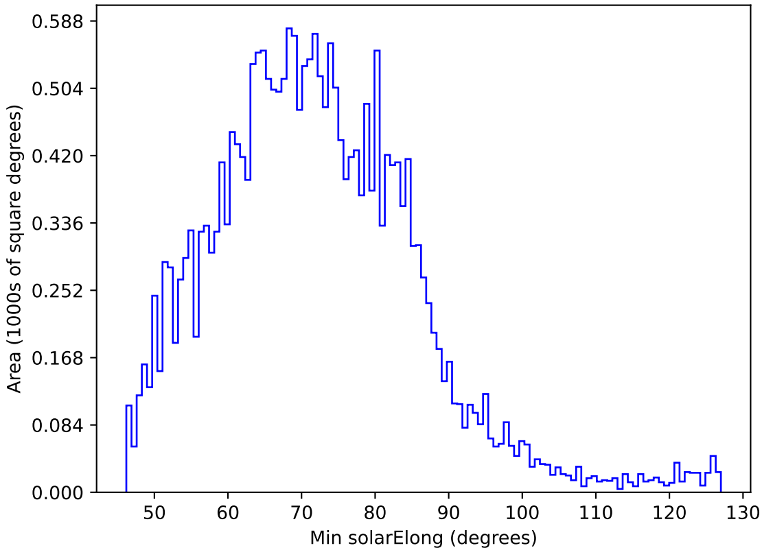
baseline_v2.0_10yrs All sky y band: Min solarElong
