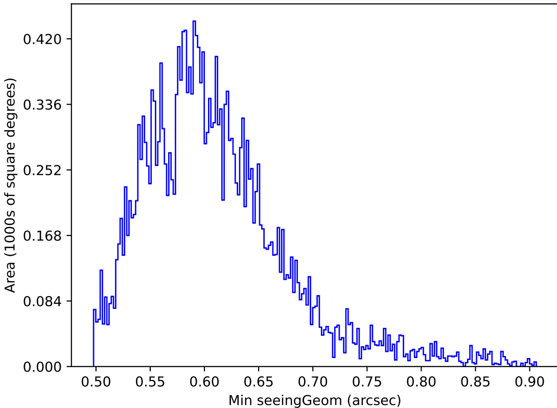
baseline_v2.0_10yrs Yr 1 y band: Min seeingGeom
