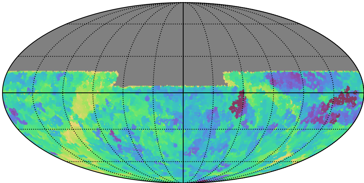
baseline_v2.0_10yrs All sky y band: Min saturation_mag
