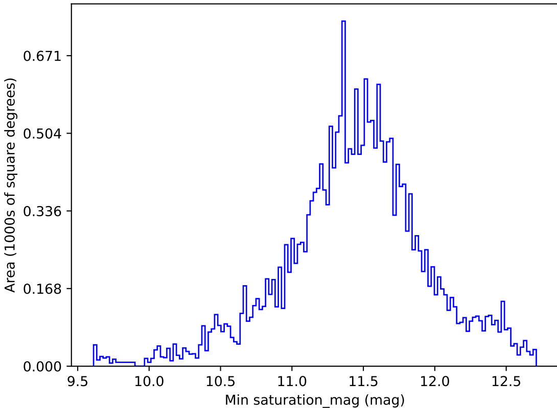
baseline_v2.0_10yrs All sky y band: Min saturation_mag
