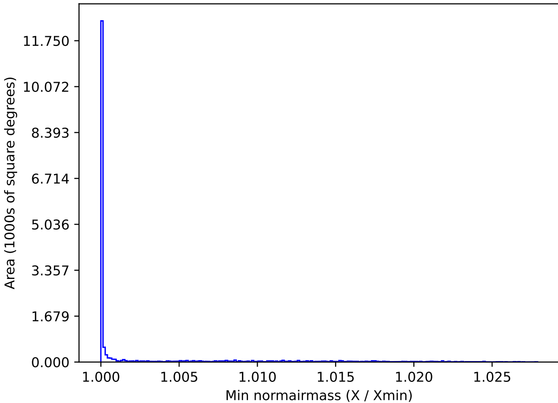
baseline_v2.0_10yrs WFD y band: Min normairmass
