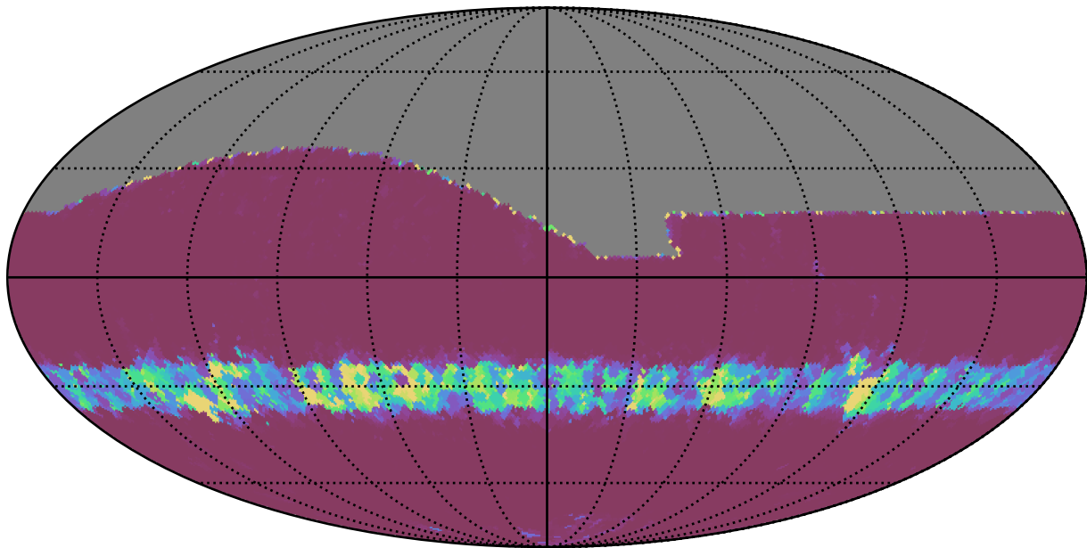
baseline_v2.0_10yrs All sky z band: Min normairmass
