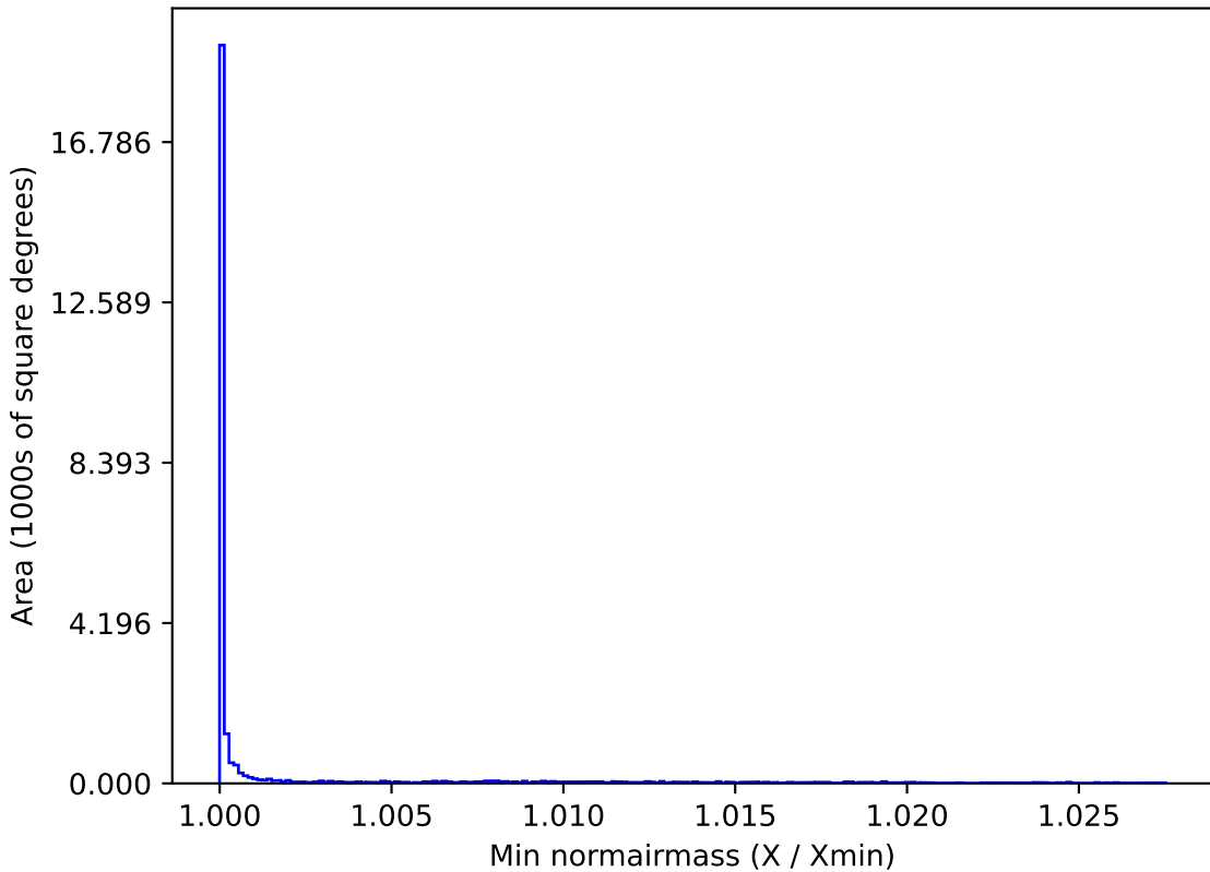
baseline_v2.0_10yrs All sky z band: Min normairmass
