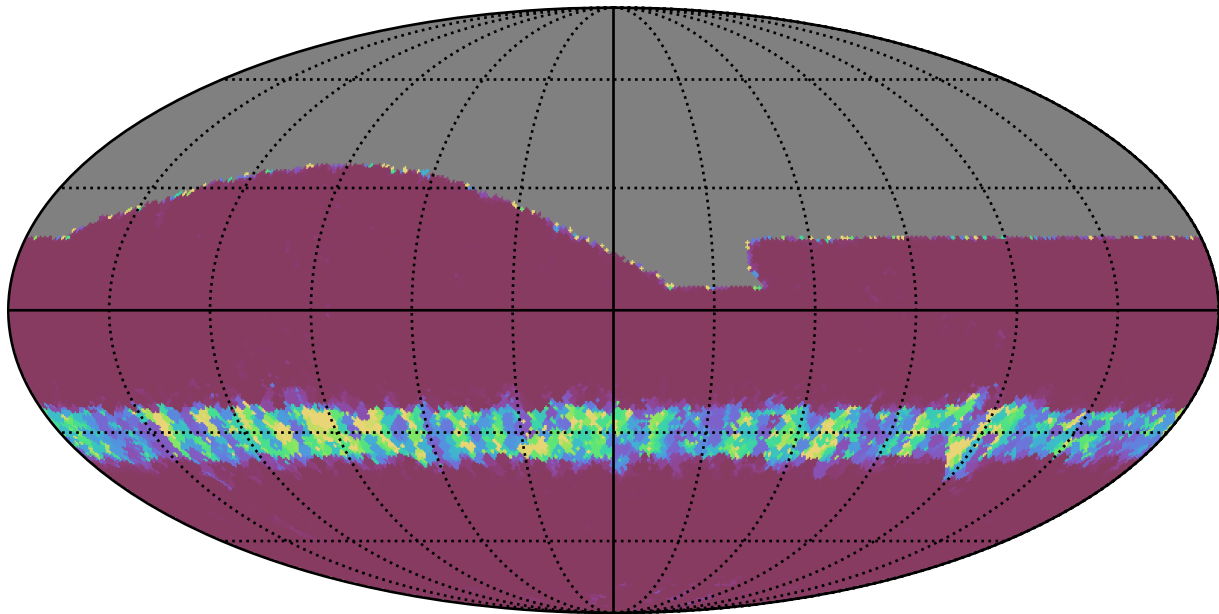
baseline_v2.0_10yrs All sky r band: Min normairmass
