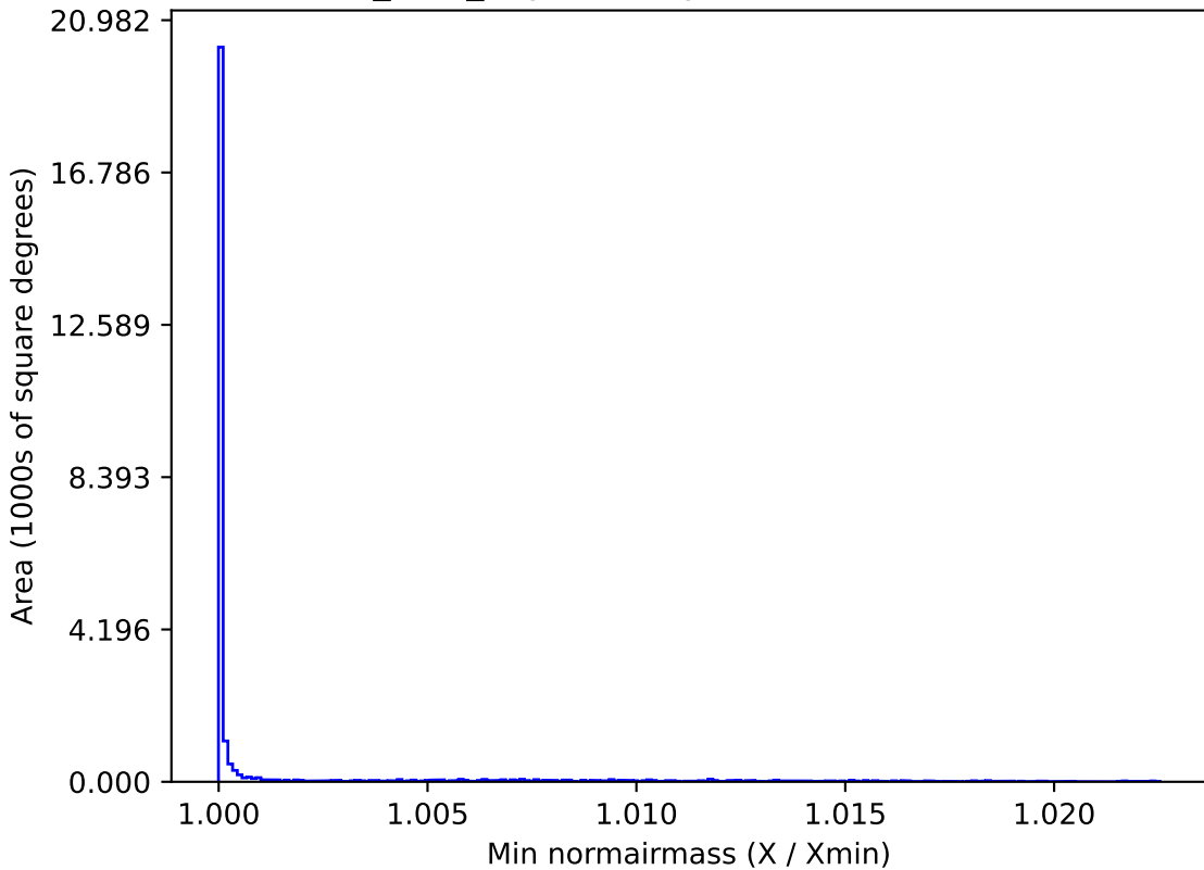
baseline_v2.0_10yrs All sky r band: Min normairmass
