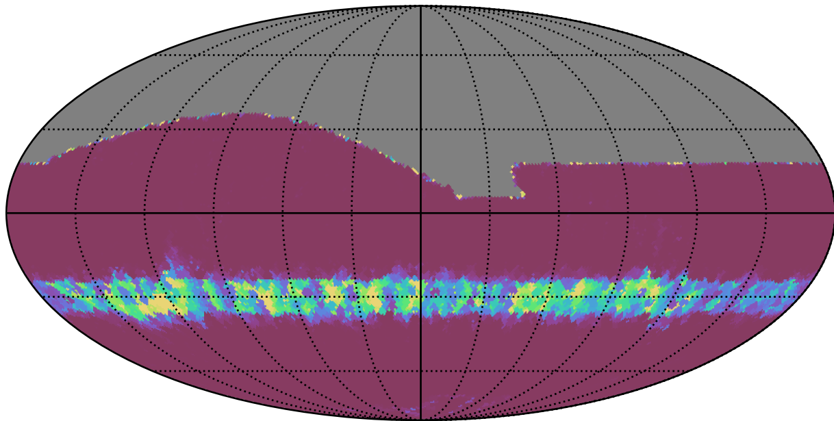
baseline_v2.0_10yrs All sky i band: Min normairmass
