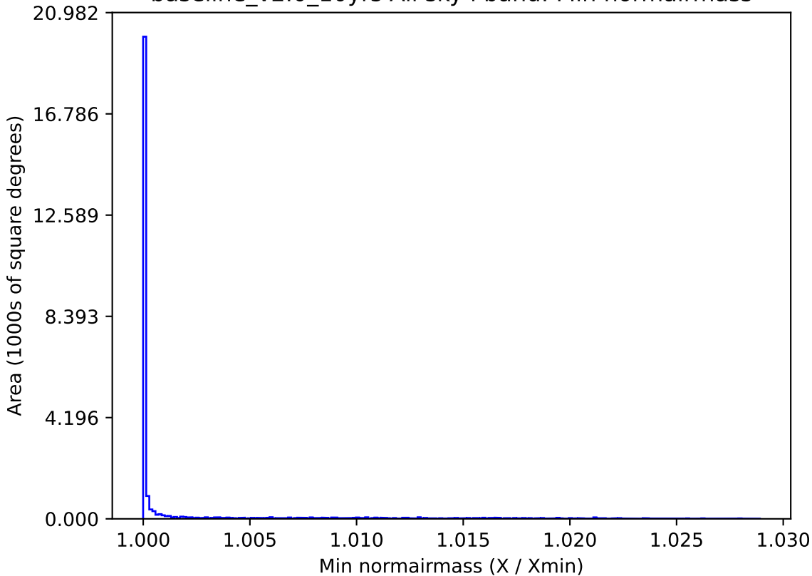
baseline_v2.0_10yrs All sky i band: Min normairmass
