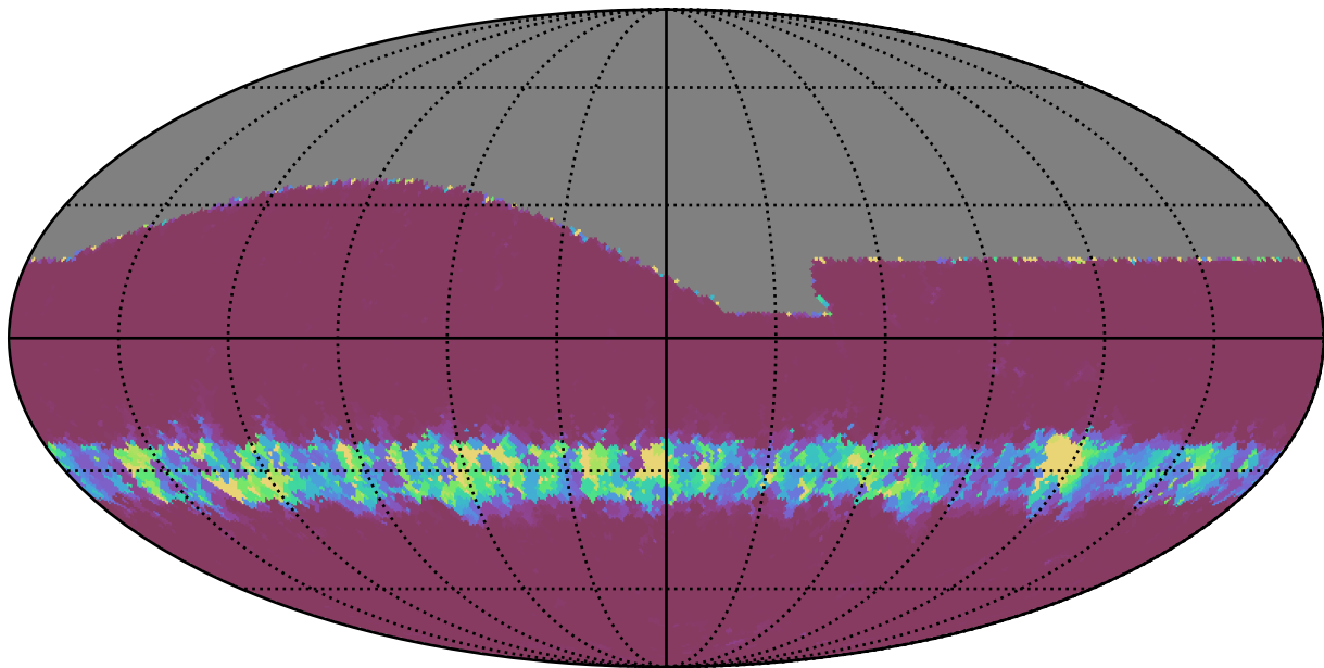
baseline_v2.0_10yrs All sky g band: Min normairmass
