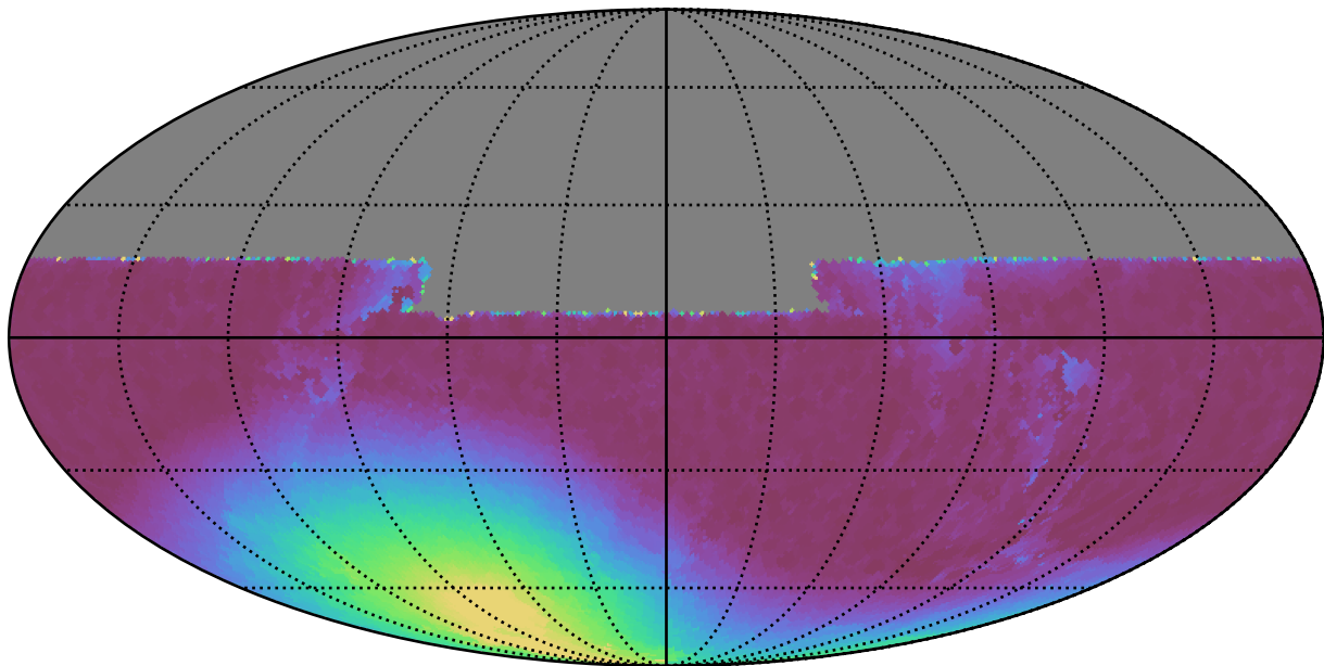
baseline_v2.0_10yrs All sky y band: Min moonDistance
